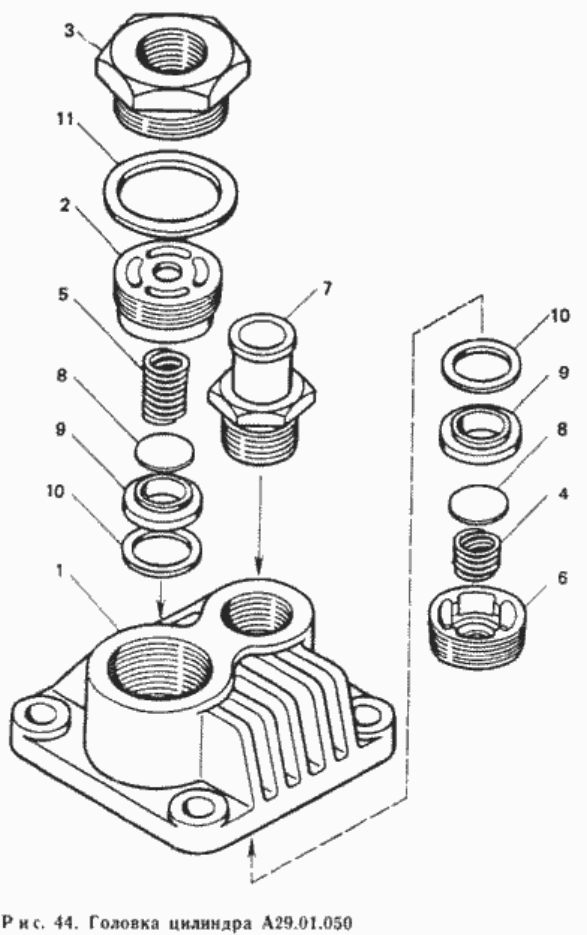
Рис. 44. Головка цилиндра А29.01.050
